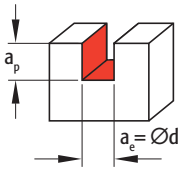
Slot milling / Nutfräsen
